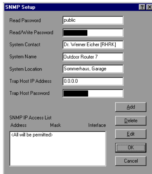
Abbildung 5.19: SNMP Daten des Routers 7
