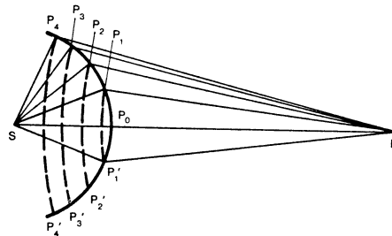
Abbildung 3.2: Beiträge zur Empfangsenergie in E
