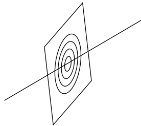
Abbildung 5.2: Die Fresnel Zonen als Kreise auf einer zur Funkstrahlausbreitungsrichtung senkrechten Fläche
