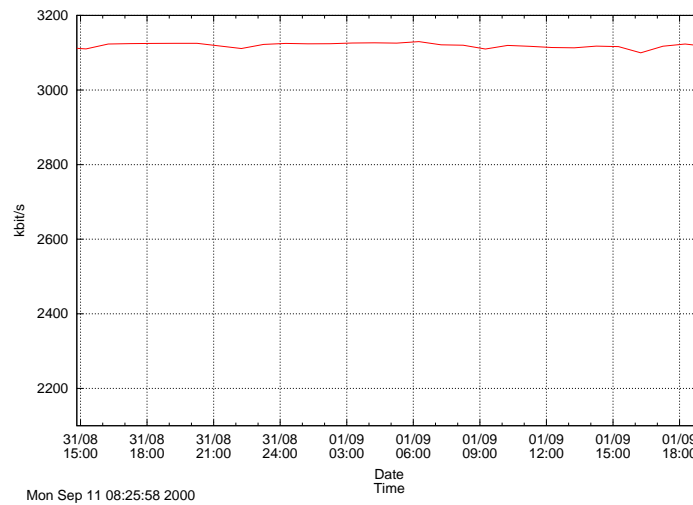
Abbildung 5.24: Resultate des Durchsatztests bei abgeschalteten Storm Thresholds mit netperf von Gebäude 7 zu dem Rechner sushi.unix-ag.uni-kl.de
