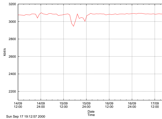
Abbildung 5.25: Resultate des Durchsatztests bei eingeschalteten Protokollfilter mit netperf von Gebäude 7 zu dem Rechner sushi.unix-ag.uni-kl.de
