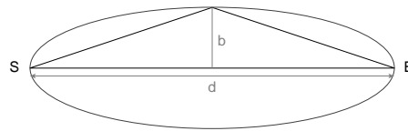
Abbildung 5.1: Erstes Fresnel-Ellipsoid zwischen Sender (S) und Empfänger (E)
