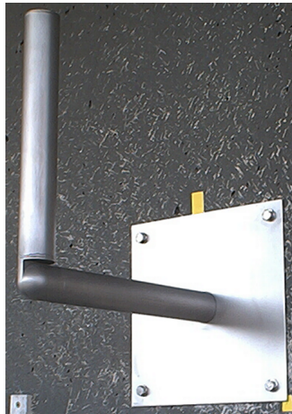
Abbildung 5.3: Der Antennenhalter an Gebäude 14
