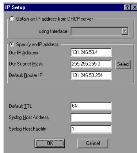
Abbildung 5.18: IP-Daten des Routers 7
