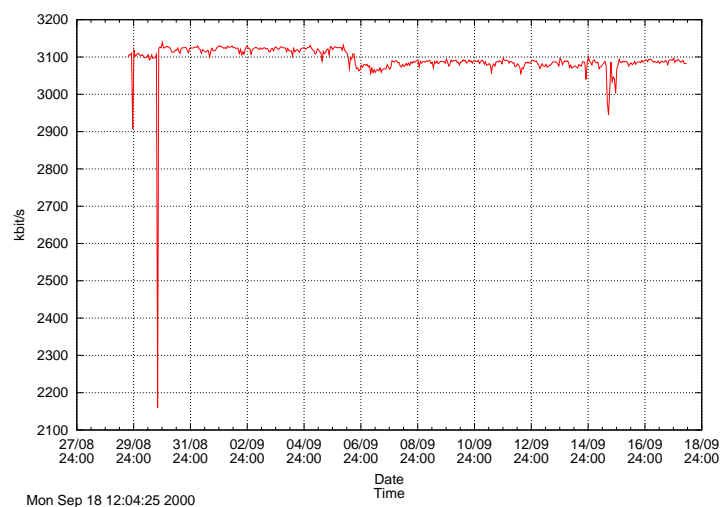
Abbildung 5.22: Entwicklung der Durchsatzrate
